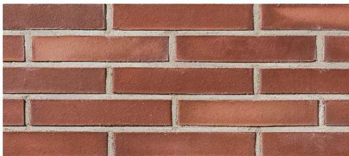
PLINFA IRON 2313 / 270x85x50 мм / пустотелый
